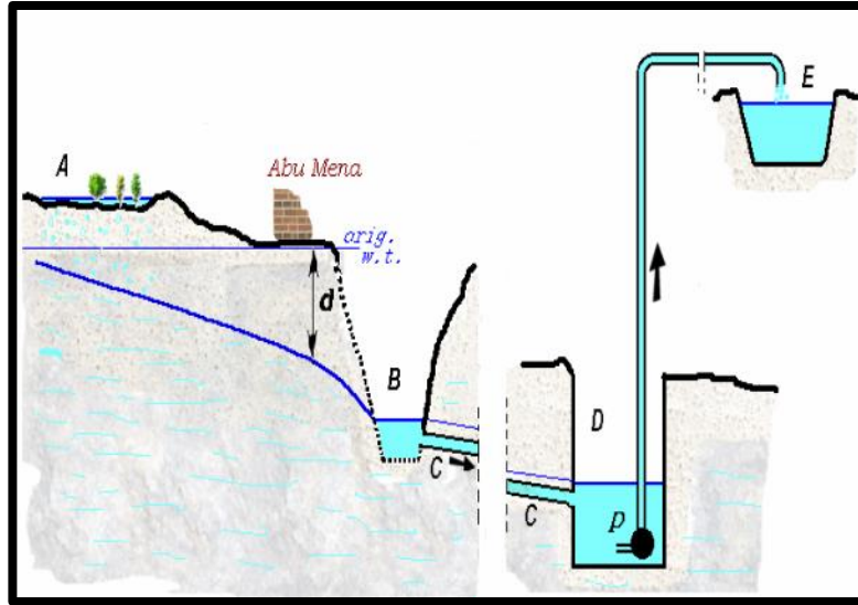
شكل (10) مشروع نقل المياه الجوفية ومياه الصرف من خلال الانابيب والمضخات بمنطقة ابومينا،
